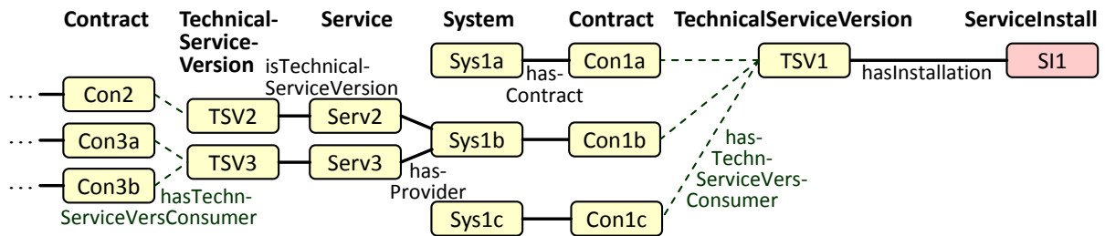
Abbildung 3: Beispieldaten aus dem SOA-Repository mit Ripple-Effect
