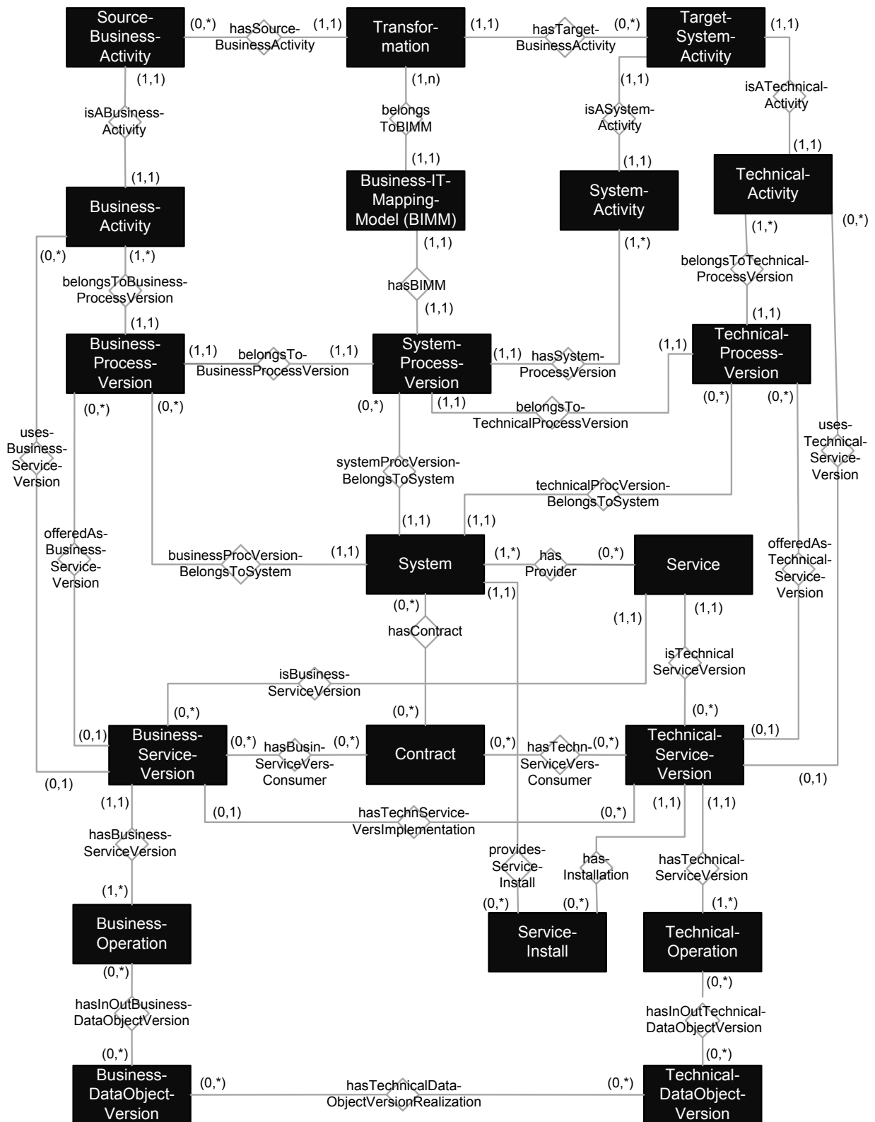
Abbildung 1: Metamodell des SOA-Repository als Entity-Relationship-Diagramm
