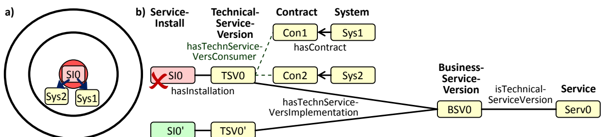
Abbildung 6: a) Impact-Graph und b) Abhängigkeiten von SI0 in 10 Monaten
